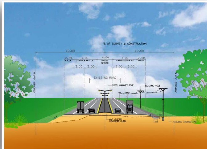
รูปแบบถนนโครงการช่วงที่ผ่านพื้นที่ชุมชน
