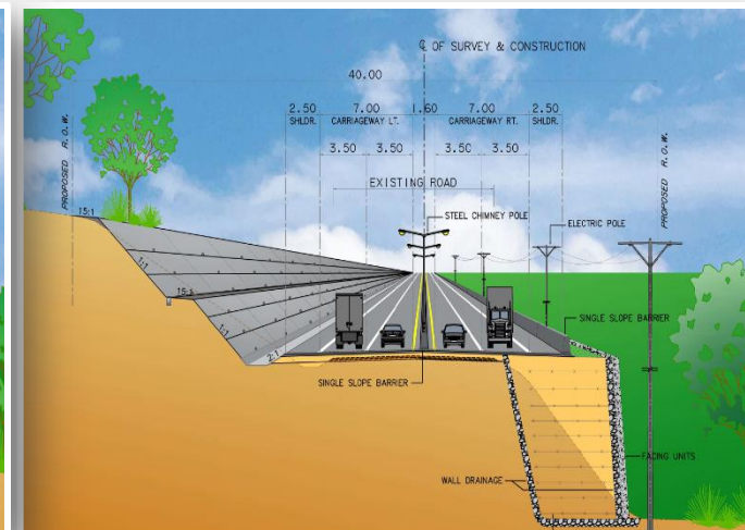
รูปแบบถนนโครงการช่วงผ่านไหล่เขาและพื้นที่ลาดชันมาก
