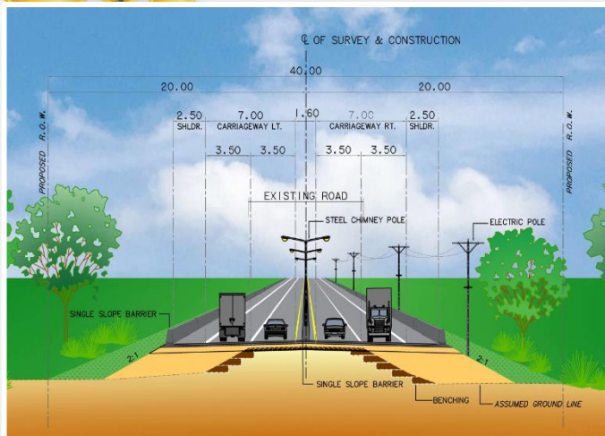
รูปแบบถนนโครงการช่วงที่ผ่านพื้นที่ทั่วไป
