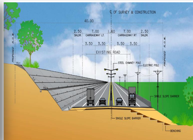
รูปแบบถนนโครงการช่วงผ่านไหล่เขาและที่ลาดชันไม่มากนัก
