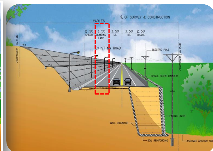
รูปแบบถนนโครงการช่วงที่ผ่านพื้นที่ลาดชันสูงหรือลึก (ในกรณีมีพื้นที่เขตทางจำกัด)
